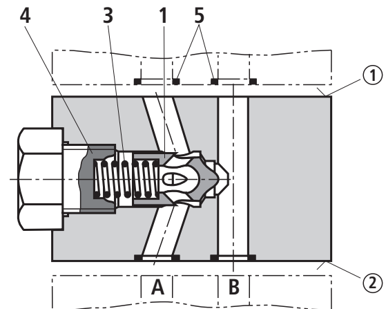
Coupe 2: Type Z1S 6 BA (vanne d'équerre)
